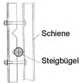
Abb. 3 Befestigung am Steigseisen
