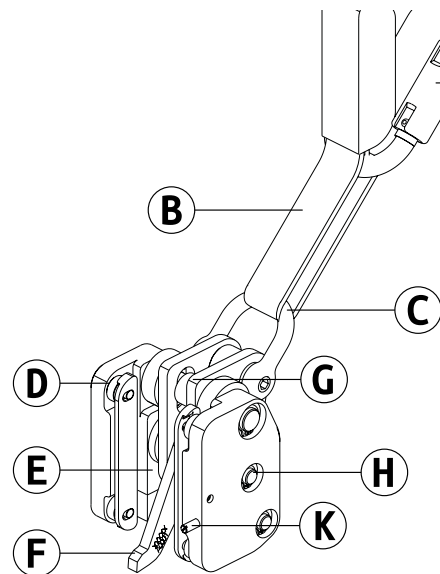
Abb. 14 Sicherungsläufer GÜFA 5
