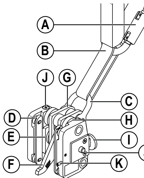
Abb. 13 Sicherungsläufer GÜFA Flexx
