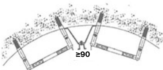
Abb. 7 Montage Steigschutzschiene zwischen Steigeisen
