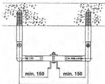
Abb. 6 Montage Steigschutzschiene an Steigeisen
