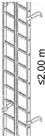
Abb. 5 Steigschutzschiene an den Sprossen einer Steigleiter bzw. Schachtleiter montiert.
