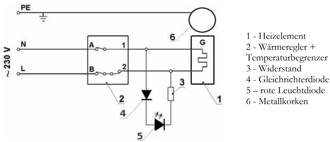
Abb. 2 Das elektrische Schema
